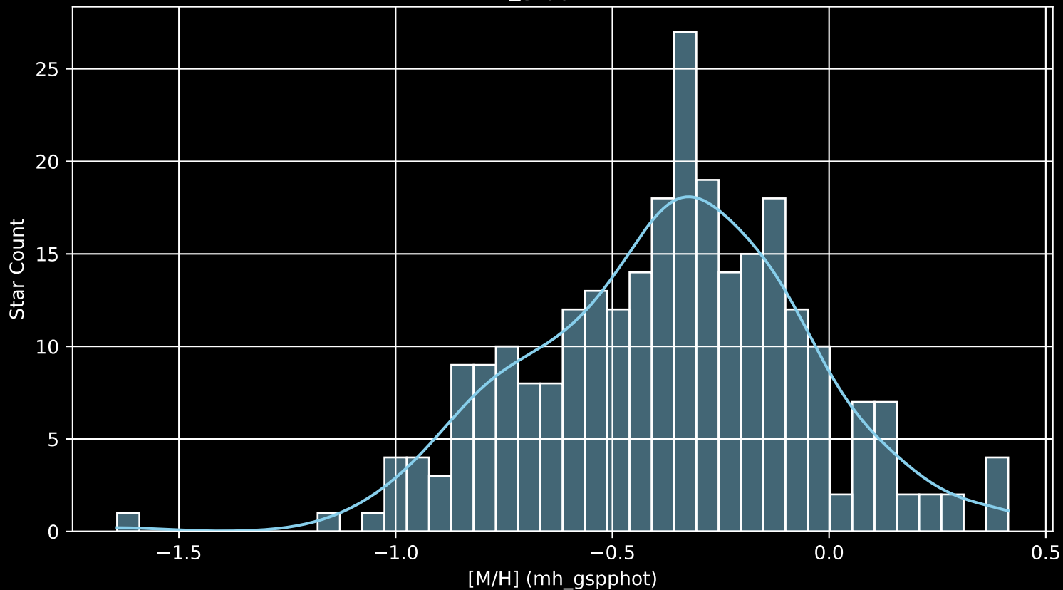
GALAH DR4 Field: [669] [M/H] (mh_gspphot) (n= 268)
