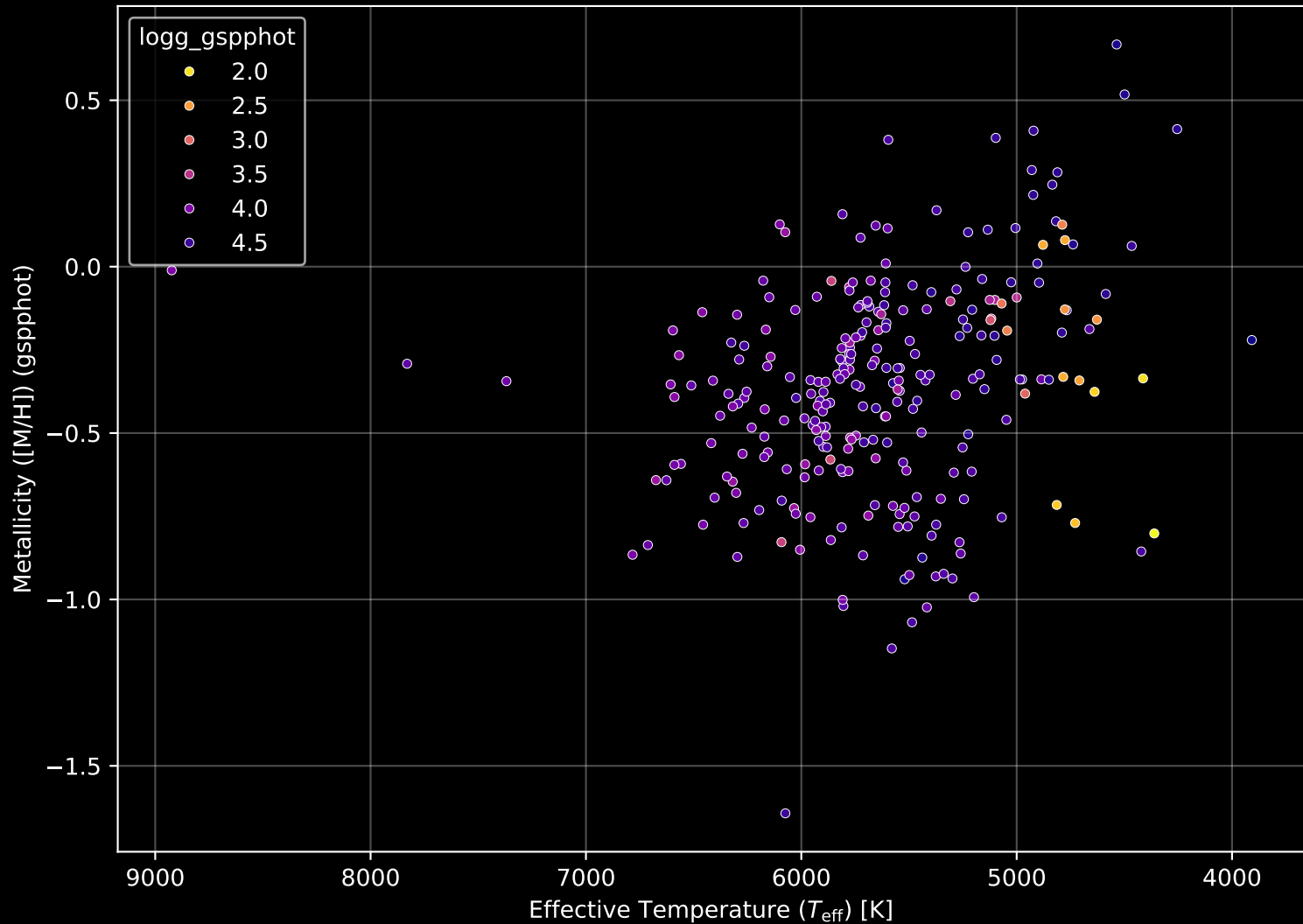
GALAH DR4 Field: [669] Stellar Population Parameters (n= 270)
