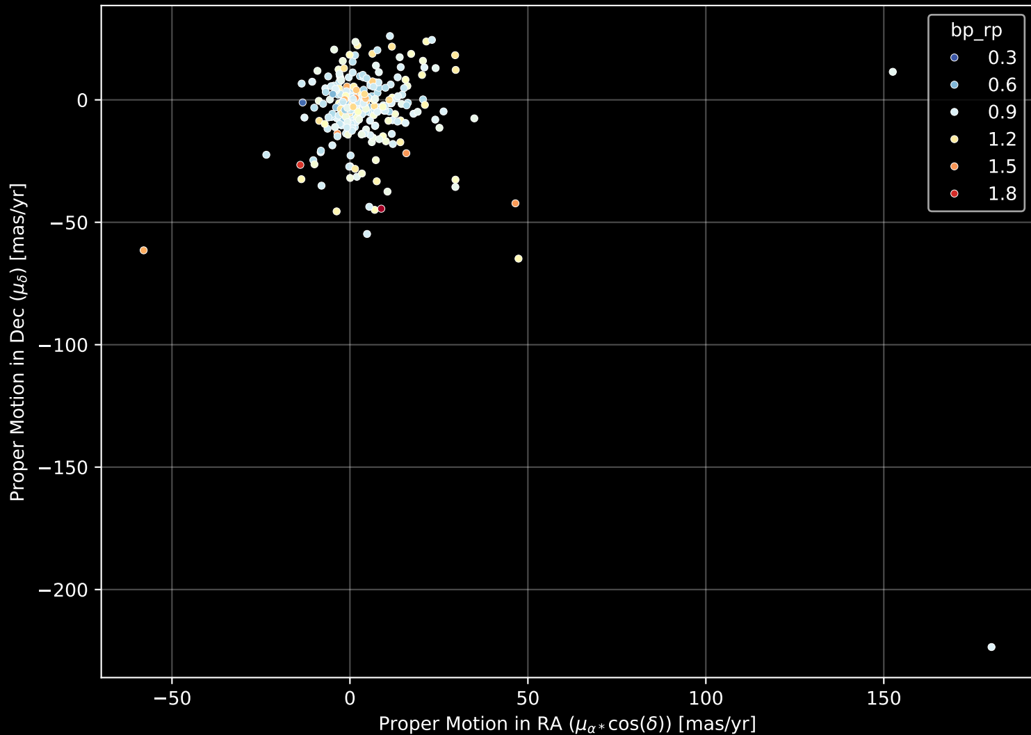
GALAH DR4 Field: [669] Proper Motion Diagram (n= 270)
