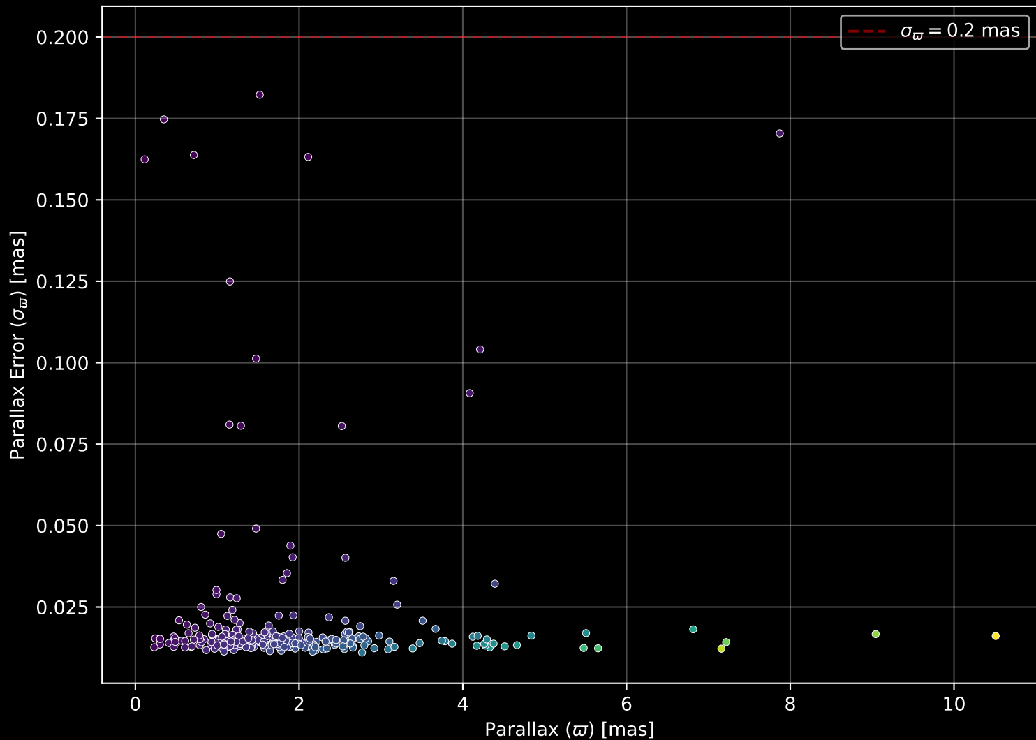
GALAH DR4 Field: [669] Parallax Quality (n= 270)
